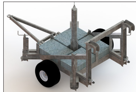
Lanzenunterbau Mobile inkl. Radsatz und Zugdeichsel
